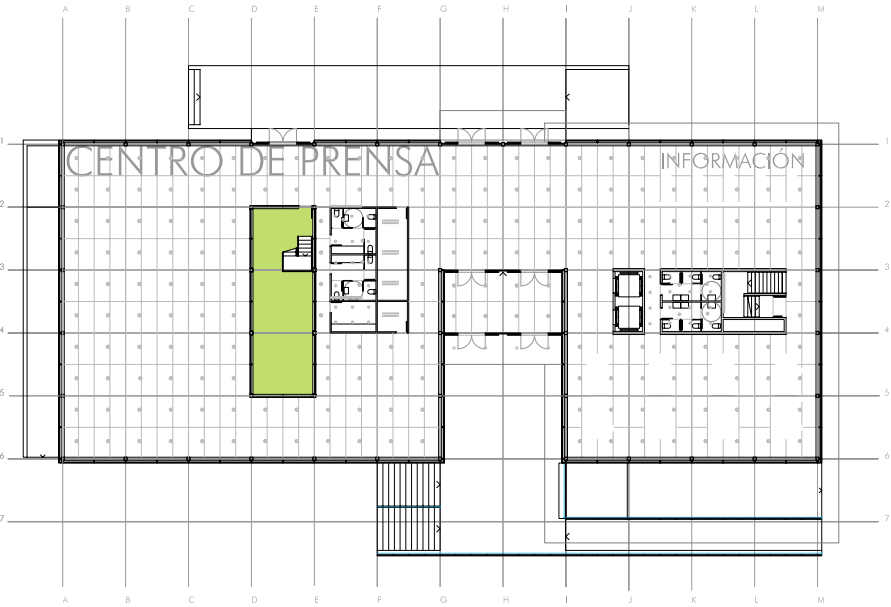
PLANTA BAJA E 1/200
