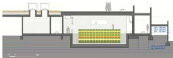
SECCIÓN S1 TRANSVERSAL
