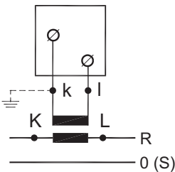
Conexión al transformador
